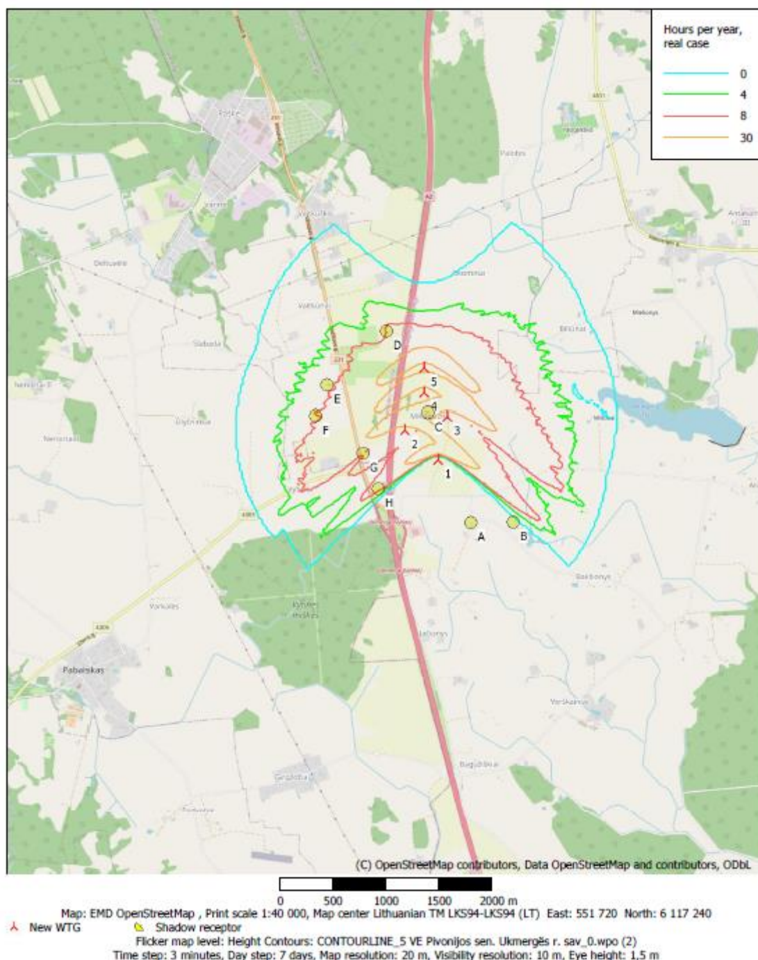
2 pav. Planuojamos Vėjo elektrinė VE-1 prognozuojamo šešėliavimo poveikio zonos sklaida
