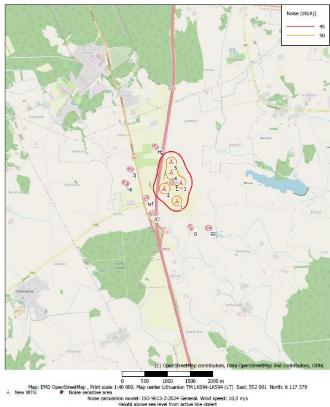
1 pav. Planuojamos Vėjo elektrinė VE-2 ir vėjo parko prognozuojamo triukšmo modeliavimo rezultatai
