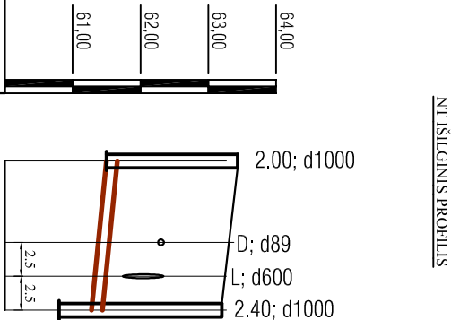
IŠILGINIS PROFILIS M h 500 v 100
