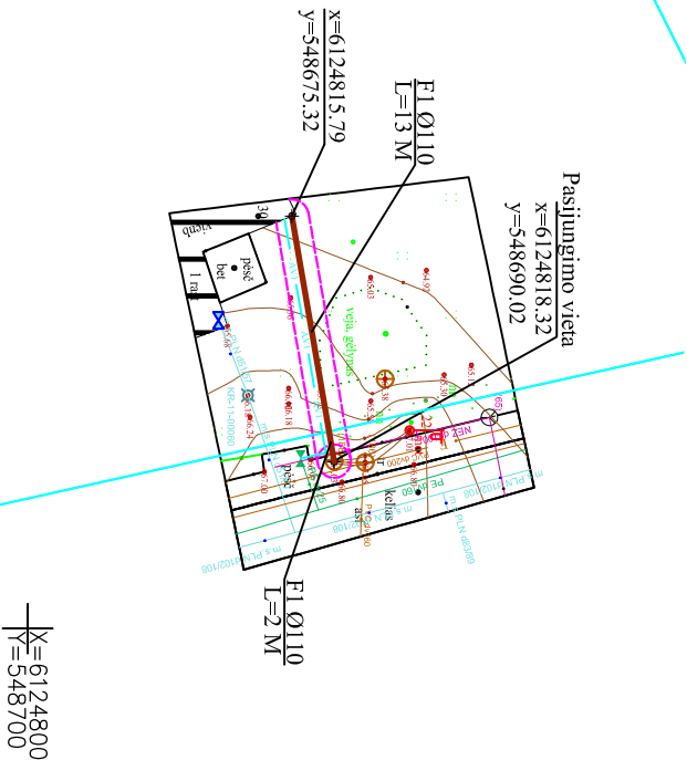
INŽINERINIŲ TINKLŲ PLANAS M 1:500
