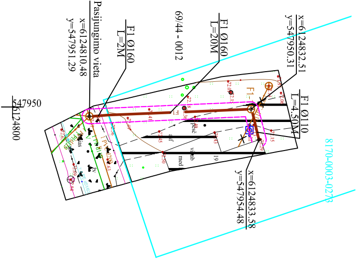
INŽINERINIŲ TINKLŲ PLANAS M 1:500
