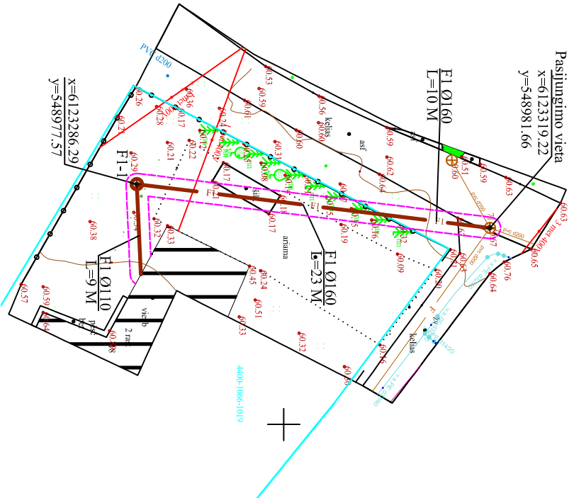
INŽINERINIŲ TINKLŲ PLANAS M 1:500
