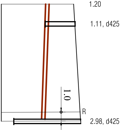
NT IŠILGINIS PROFILIS
