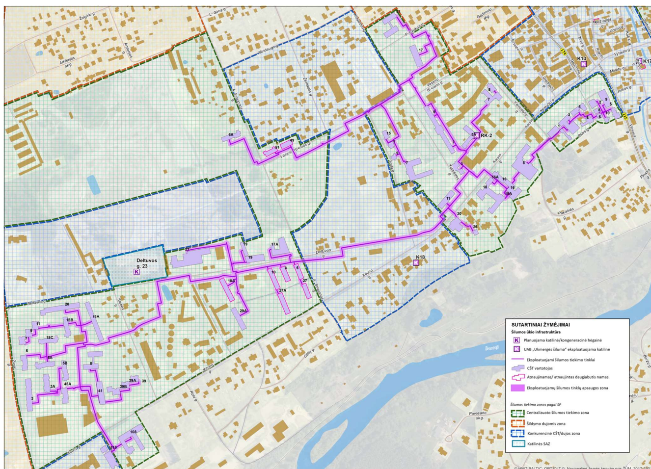
5-4 pav. RK-2 katilinės centralizuoto šilumos tiekimo sistemos schema
