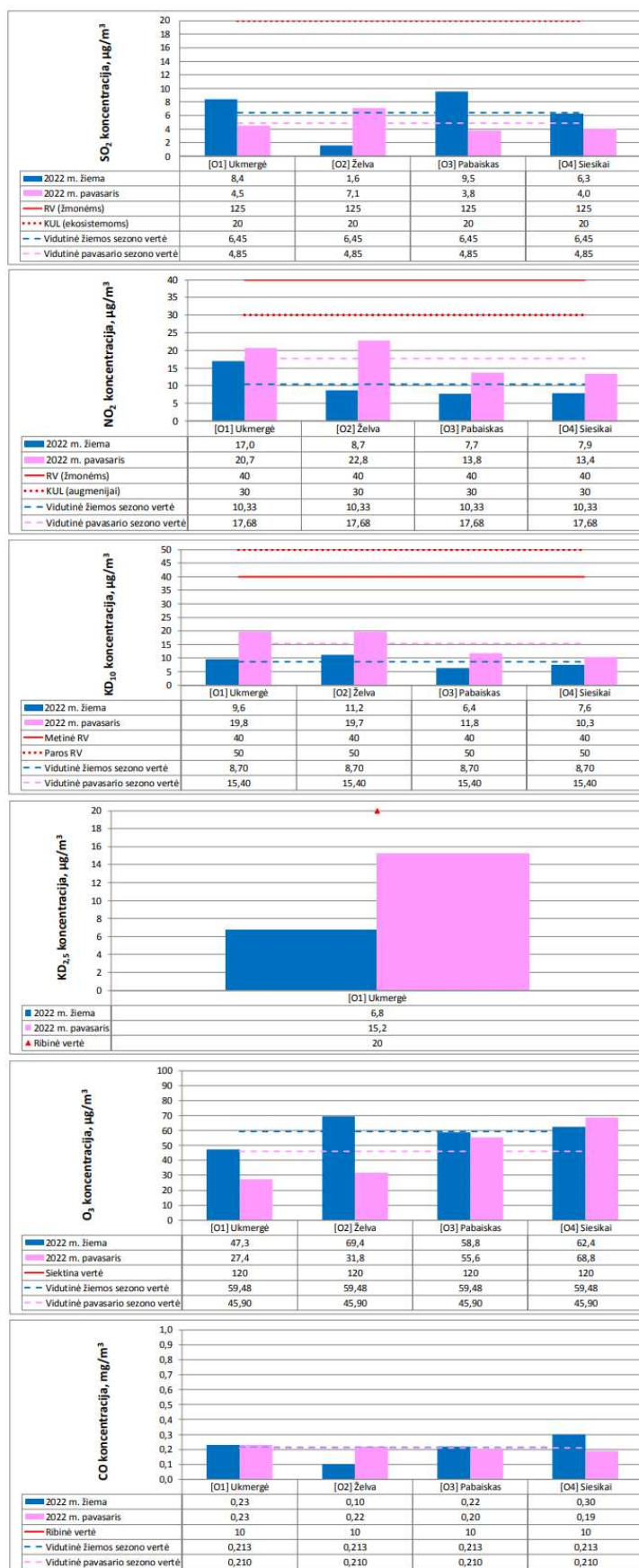
7-1 pav. Oro teršalų koncentracijos aplinkos ore Ukmergės rajone (duomenų šaltinis: Aplinkos monitoringo programos įgyvendinimo paslaugos ataskaita už 2022 metų I pusmetį)
