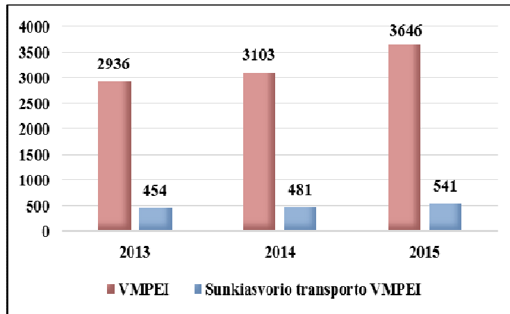
8 pav. Vidutinis metinis paros eismo intensyvumas (VMPEI) magistraliniuose ir krašto keliuose 2013–2015 m., apskaičiuotas įvertinant aritmetinį svertinio VMPEI vidurkį pagal KTTI duomenis.
